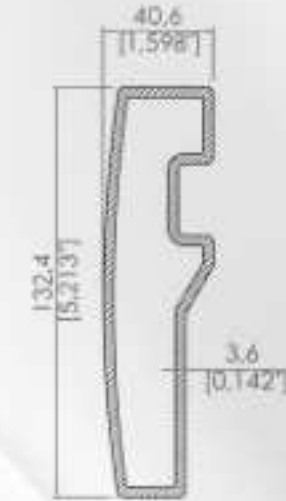
40,6x132,4 Oluk Eki Profili 40,6x132,4 Gutter Profile Connection
