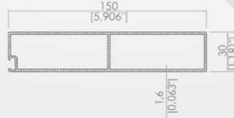
30x150 Kutu Profili 30x150 Box Profile
