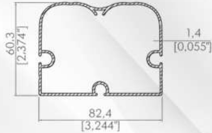
82,4x60,3 Kalın Korniş 82,4x60,3 Fabric Support Profile
