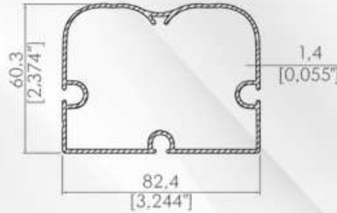
82,4x60,3 Kalın Korniş 82,4x60,3 Fabric Support Profile
